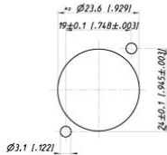
Frontplatten-Ausschnitt (von hinten)
